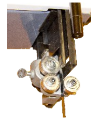
Kugelgelagerte Bandführung
