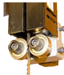
Bandführung oben
