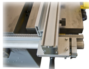
Exakter Parallelanschlag
