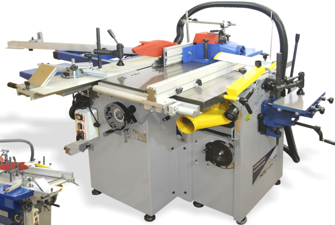
massiver Formatschiebeschlitten
